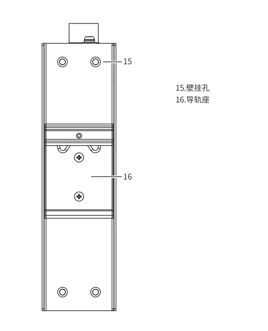
TL-SG2206R工业级 后面板示意图
