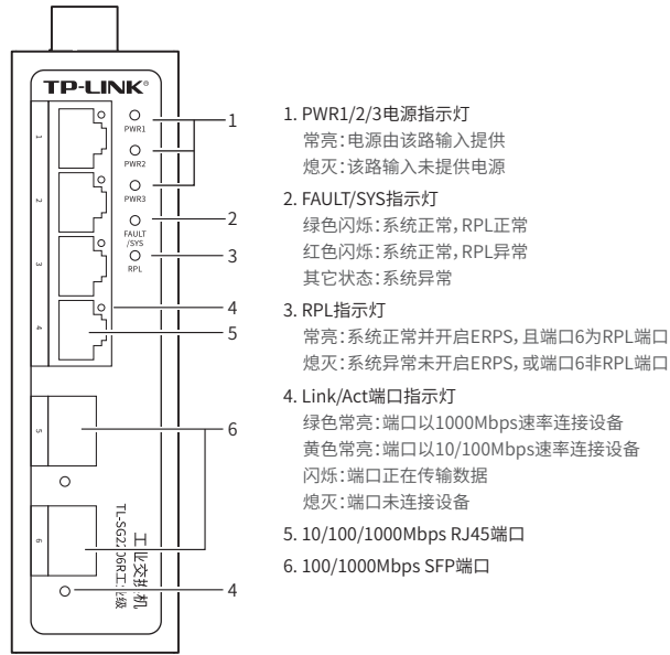
TL-SG2206R工业级 前面板示意图
