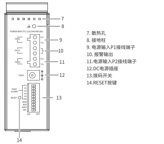
TL-SG2206R工业级 上面板示意图
