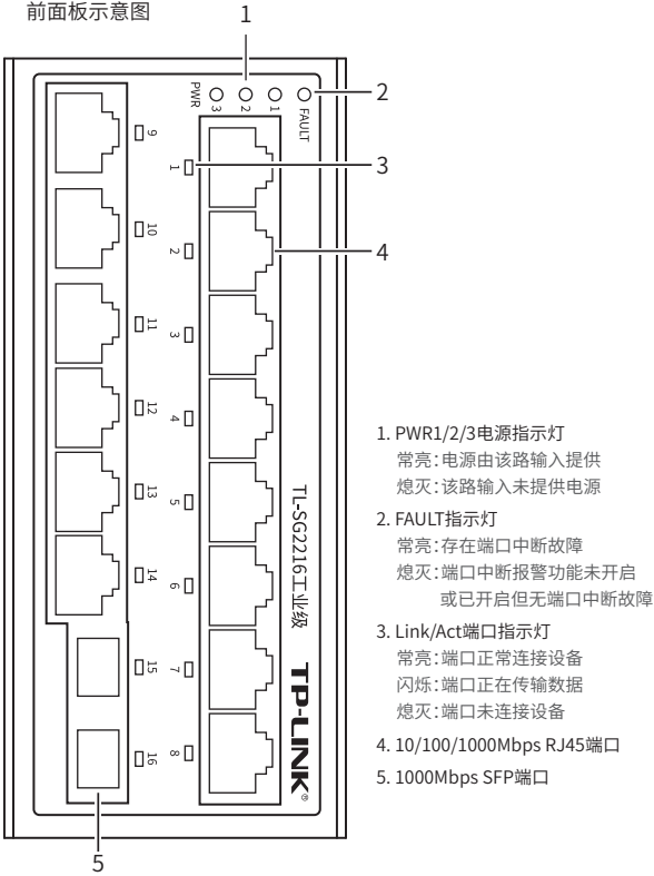
TL-SG2216工业级 前面板示意图
