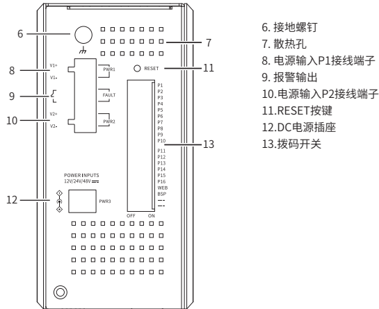
TL-SG2216工业级 上面板示意图
