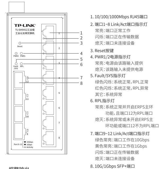
TL-SH5412工业级前面板示意图
