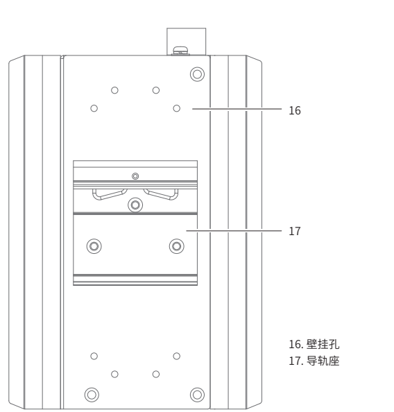
TL-SH5412工业级后面板示意图
